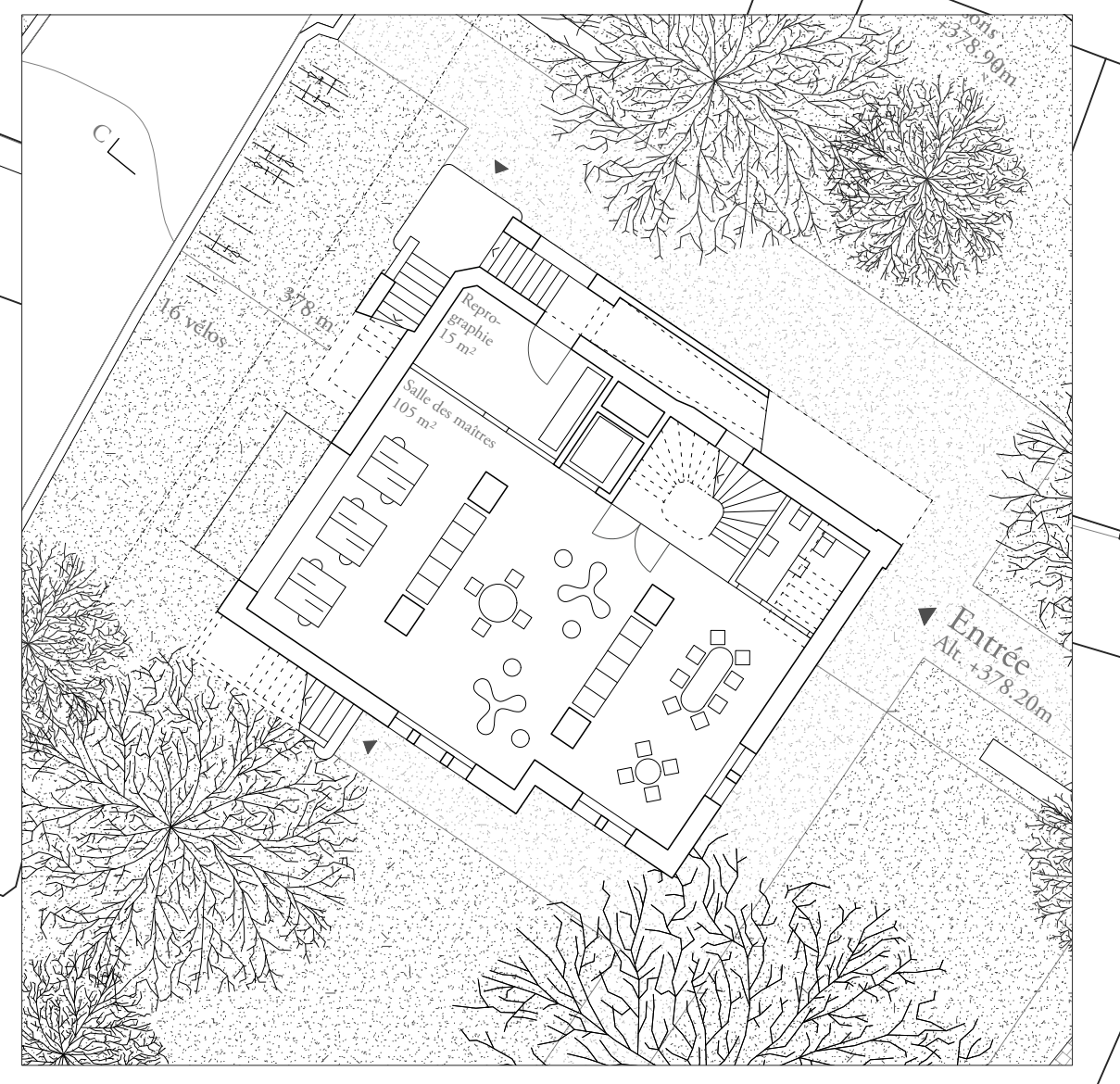
Plan du rez-de-chaussée inférieur | 1:200
